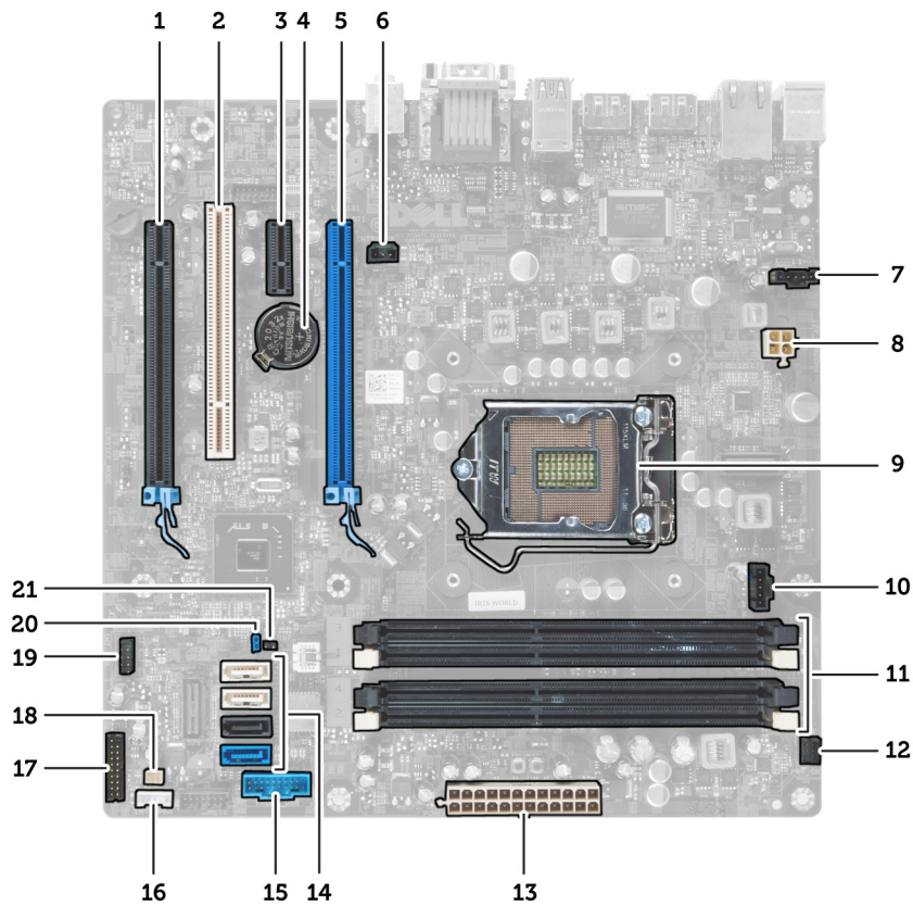
图 1: 系统板组件
